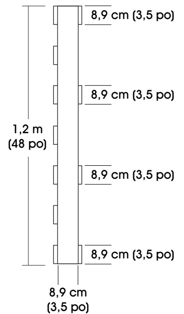
VUE LATÉRALE
