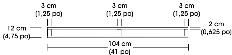
VUE LATÉRALE
